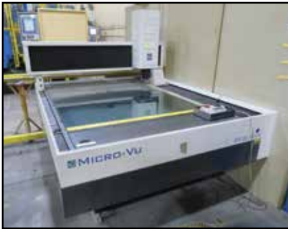
MICRO VU Excel 1051 UM Lamina CMM
